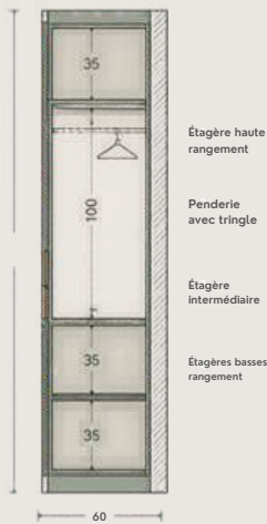
COUPE LATÉRALE
