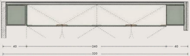
PLAN (VUE DE DESSUS)
